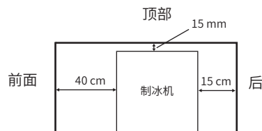
侧视图
